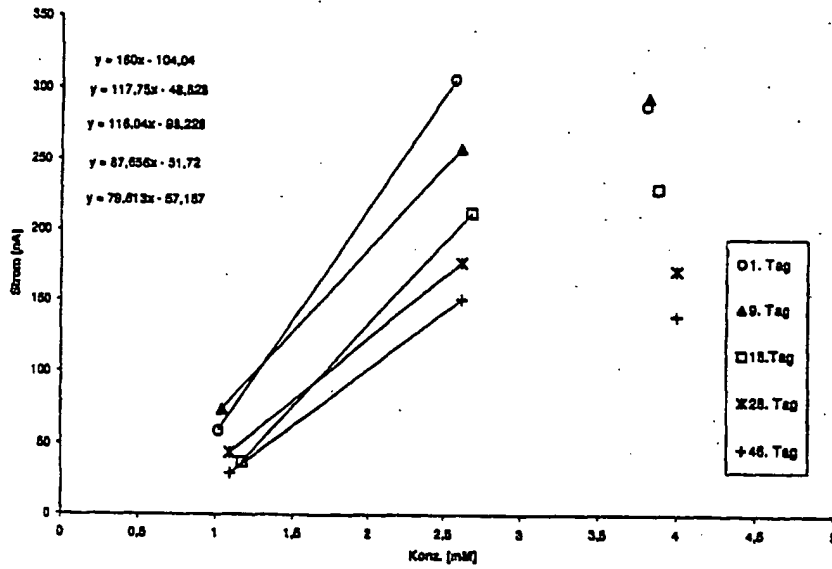
Abbildung 13: Sensitivität von TMPD-modifizierten Glukosebiosensoren ohne Schutzschicht in Abhängigkeit des Sensoralters
